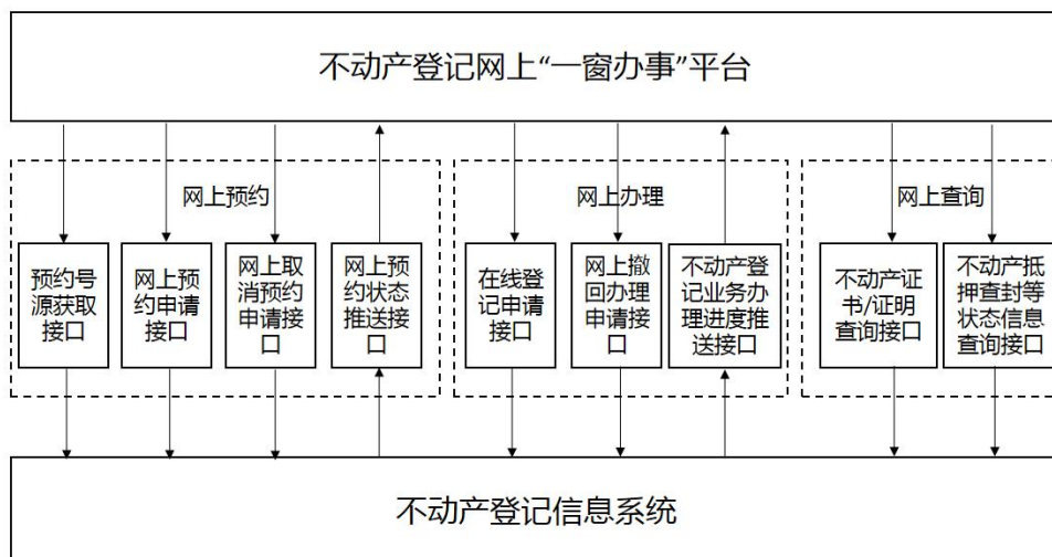
图 1 接口构成图
